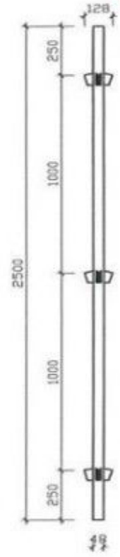
GIÀN NÊM L=2500mm
